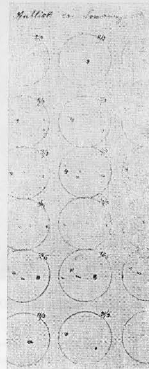
Из метеорологических тетрадей — схемы расположения солнечных пятен.
